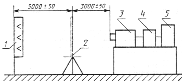
1 - экран; 2 - держатель образцов; 3 - телевизионная установка; 4 - электронное устройство; 5 - частотомер Черт. 5
