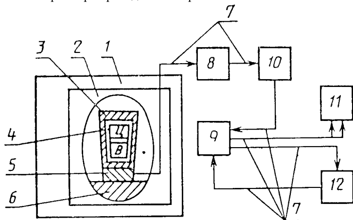
1-термостат; 2 - калориметрический блок; 3 - камера; 4 - ячейка; 5 - тепломер; 6 - теплоотвод; 7 - соединительные кабели; 8 - коммутатор; 9 - калибратор; 10 - предварительный усилитель; 11 - самописец; 12 - интегратор
