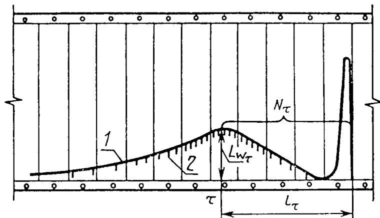
1 - кривая отклонения пера самописца; 2 - сброс пера самописца
